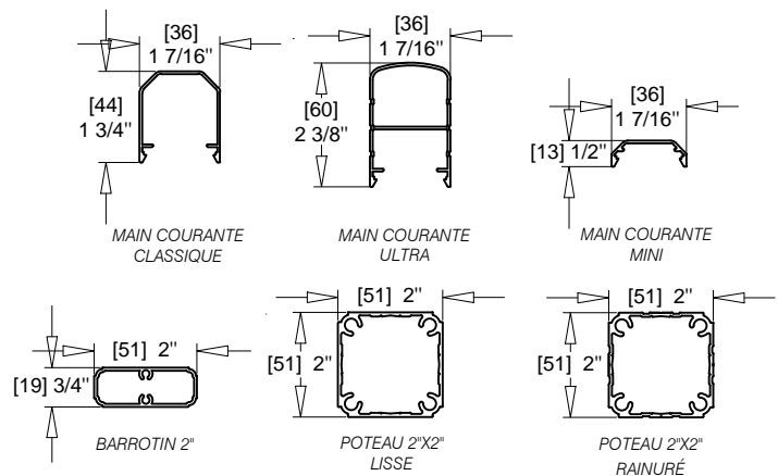
DÉTAILS | ÉCHELLE: 1:4
