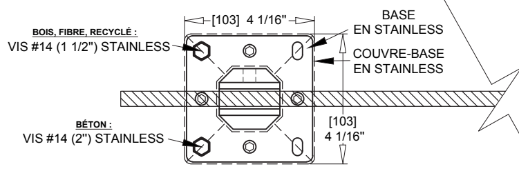
VUE EN PLAN | ÉCHELLE: 1:4
