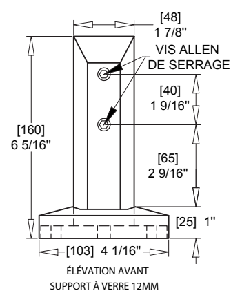
DÉTAILS | ÉCHELLE: 1:4
