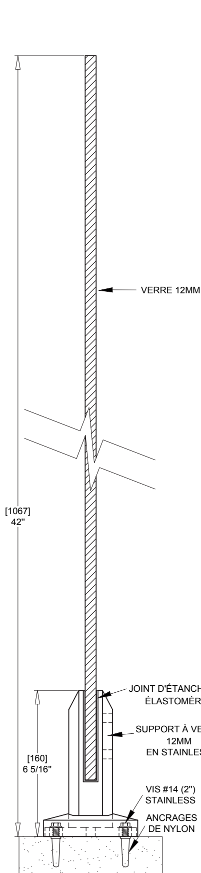
COUPE TYPE | ÉCHELLE: 1:4
