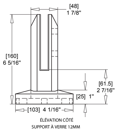
DÉTAILS | ÉCHELLE: 1:4
