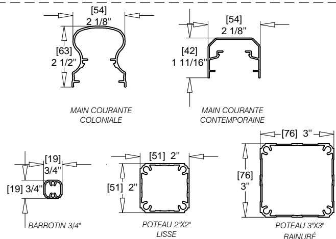
DÉTAILS | ÉCHELLE: 1:4
