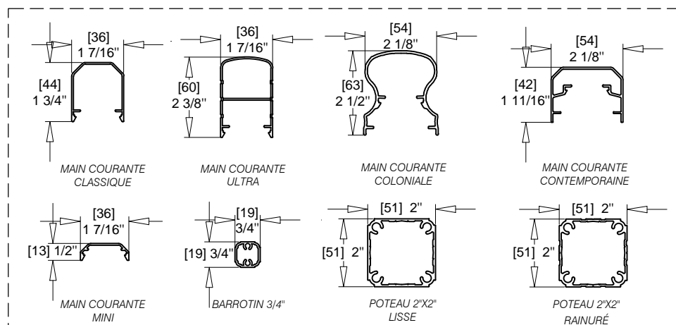
DÉTAILS | ÉCHELLE: 1:4
