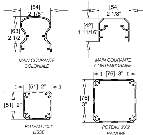
DÉTAILS | ÉCHELLE: 1:4
