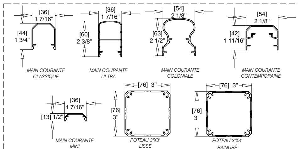
DÉTAILS | ÉCHELLE: 1:4
