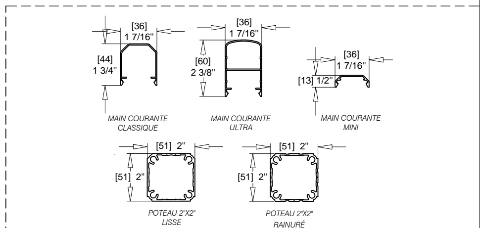
DÉTAILS | ÉCHELLE: 1:4
